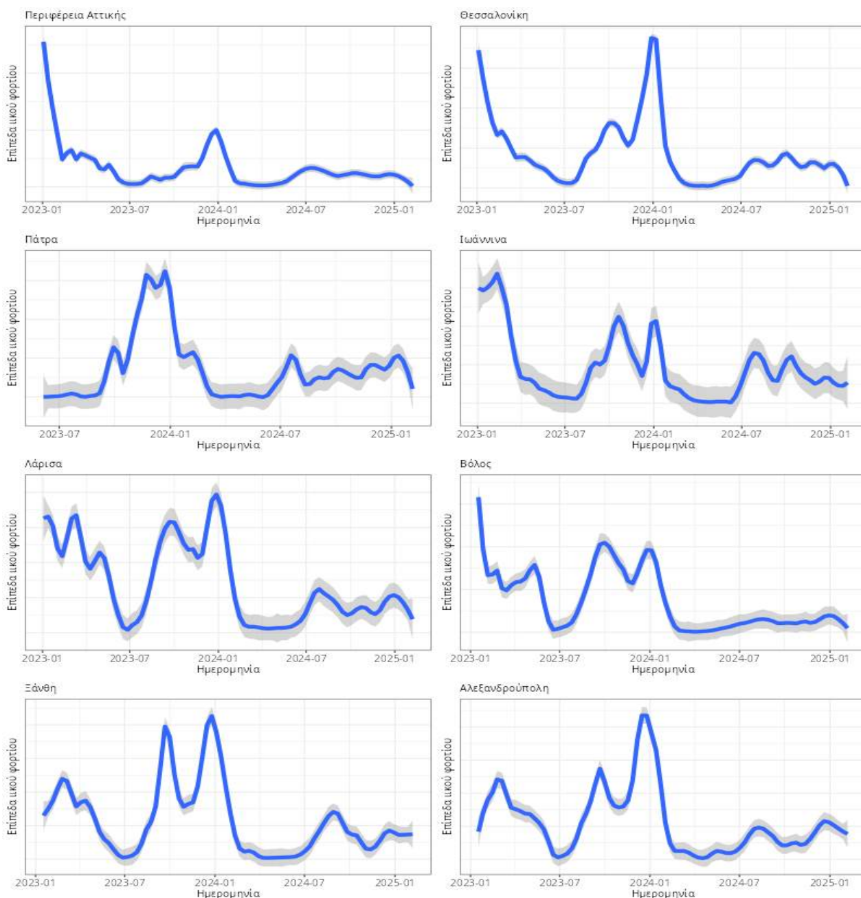
Διάγραμμα 18: Διακύμανση επιπέδων ιικού φορτίου (γονιδιωματικά αντίγραφα/100.000 πληθυσμό) στα αστικά λύματα συναρτήσει του χρόνου κατά την περίοδο 01/01/2023-09/02/2025
